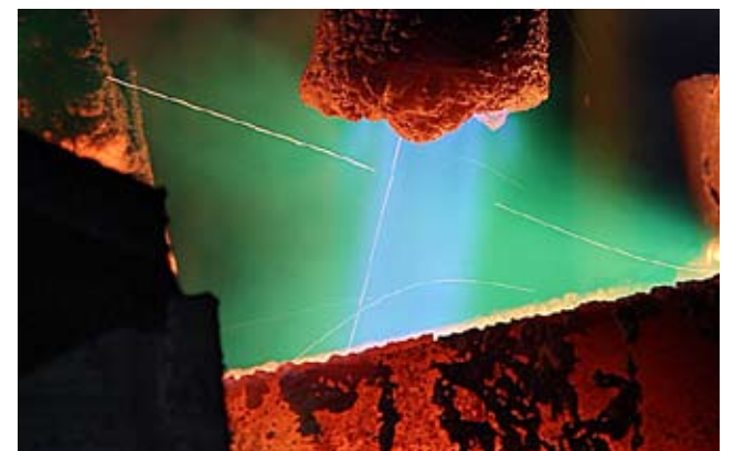
Huta Miedzi Cedynia - linia ciągłego odlewu walcówki
